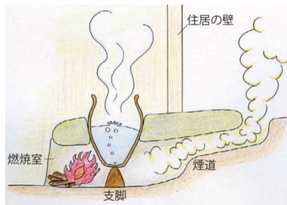
カマドの構造 長野県埋蔵文化財センター 2005『三角原遺跡』
