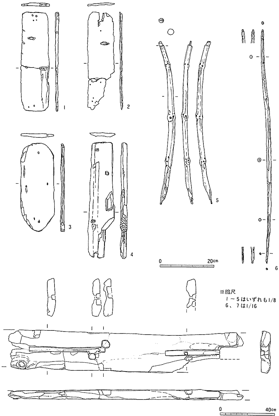
第42図 川田糸里遺跡出土の木製品実測図（1～4、田下駄 5・6、弓 7、建築部材）
