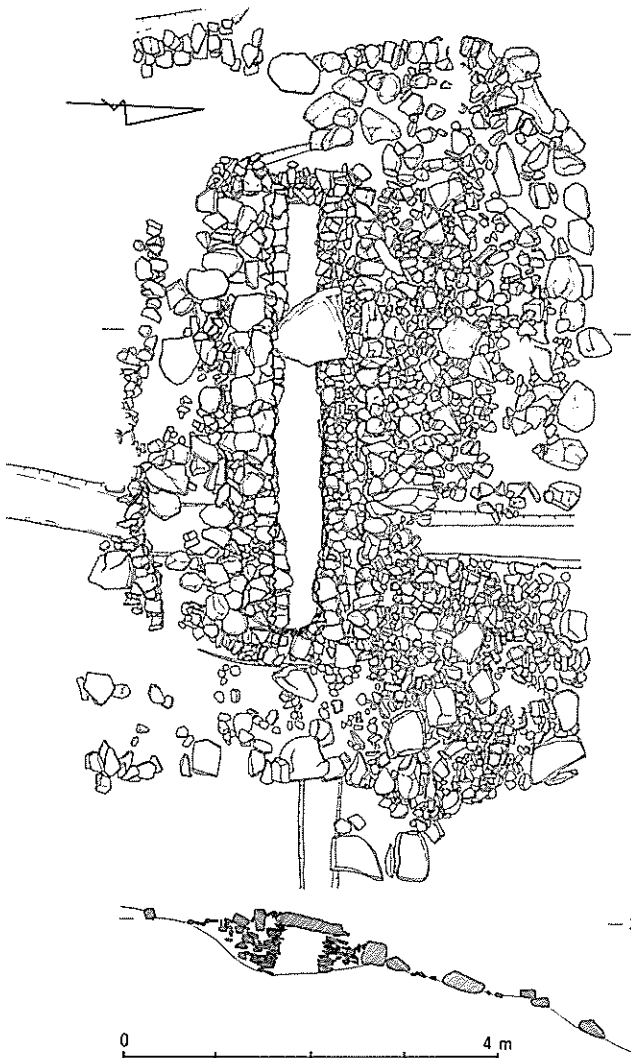
第47図 大星山4号墳の石室平面図(1:100)
