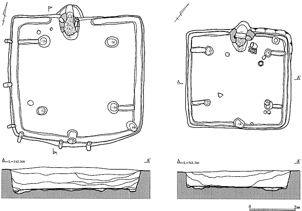
第67図 長土呂遺跡群の36・49号住居跡実測図(1:100)
