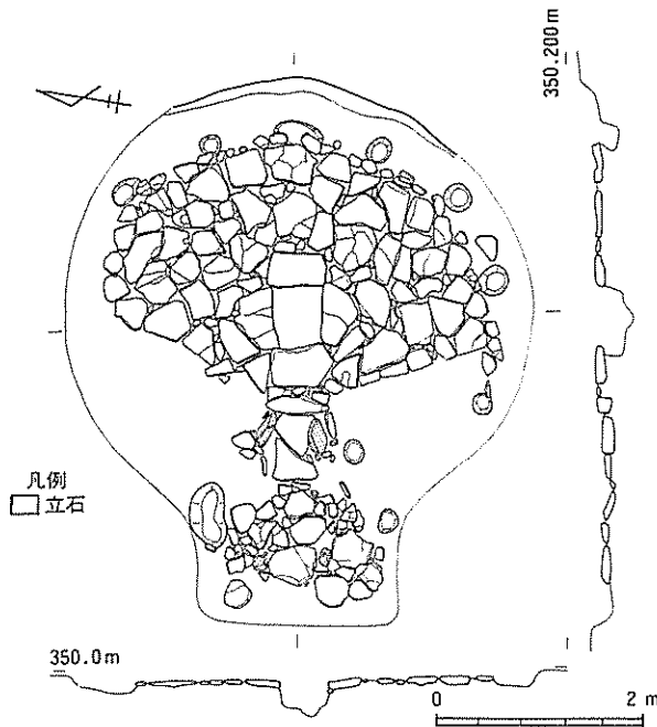
第29図 村東山手遺跡 8号敷石住居跡 (1:80)
